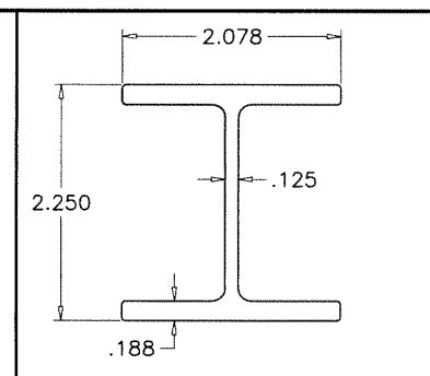
ASTRAGAL STIFFENER
