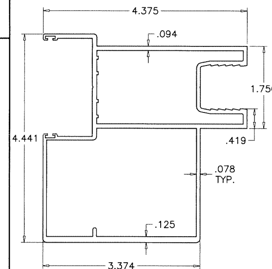
ASTRAGAL STILE (LAM. GLASS)
