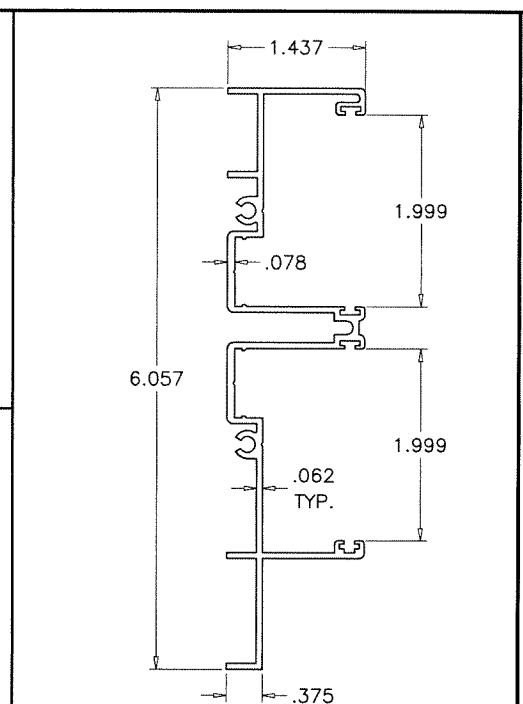
FRAME JAMB
